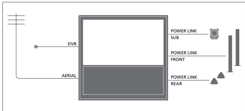
Opstelling BeoVision 10-40/46
